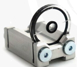
Kornhalter mit Ringkorn und Kontrollring
