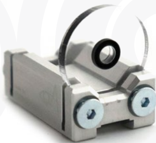
Kornhalter mit Ringkorn
